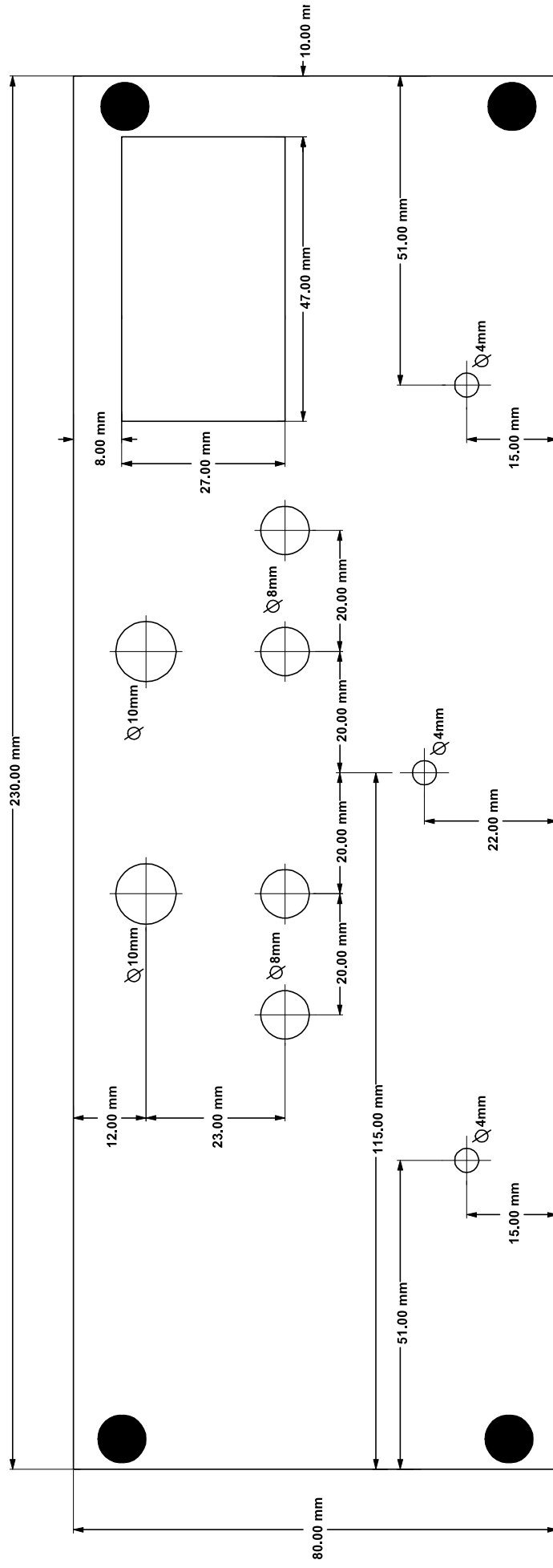
Pannello posteriore (vista retro mobile) Piano foratura
