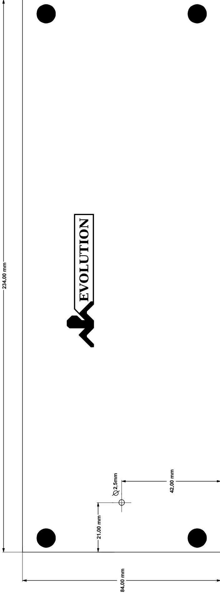
Pannello anteriore (vista frontale)
