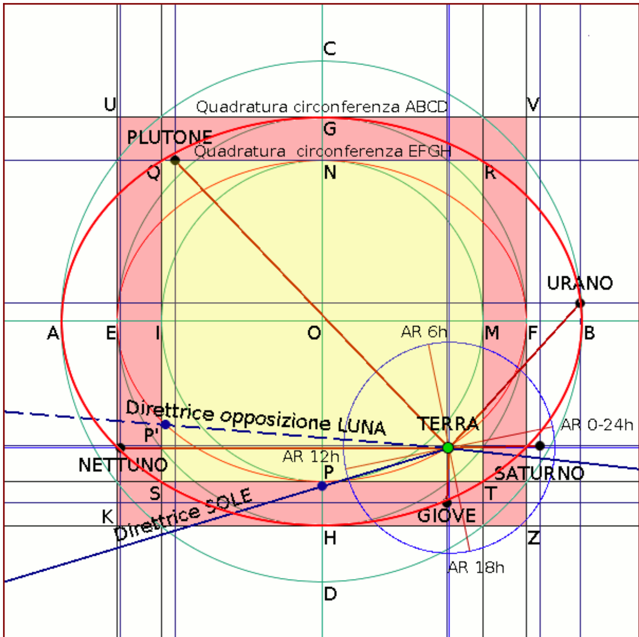
Illustrazione 2: Astro-geometria solare dei pianeti lenti.
